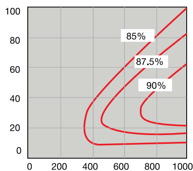
Эффективность DC-мотора
